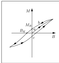
Abbildung 11.18: Hysteresekurve eines Ferromagneten.
