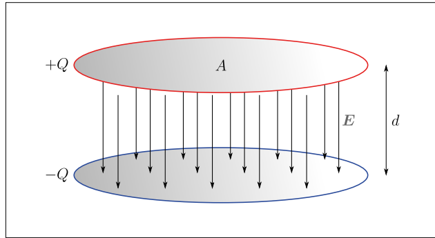
Abbildung 3.8: Ein Plattenkondensator.
