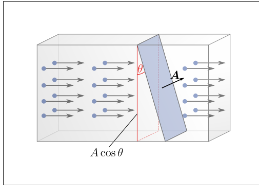
Abbildung 4.2: Zusammenhang zwischen Stromdichte und Stromstärke.
