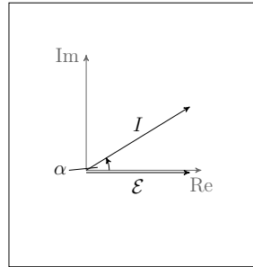
(b) Repräsentation im Zeigerdiagramm. Der Strom eilt der Spannung voraus.
