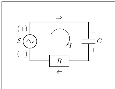
(a) Einfacher RC -Stromkreis. Eine momentane Stromrichtung (Polarität von \mathcal{E} in Klammern) ist eingezeichnet.
