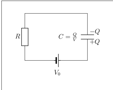
Abbildung 4.6: Schaltbild für die Ladung eines Kondensators.
