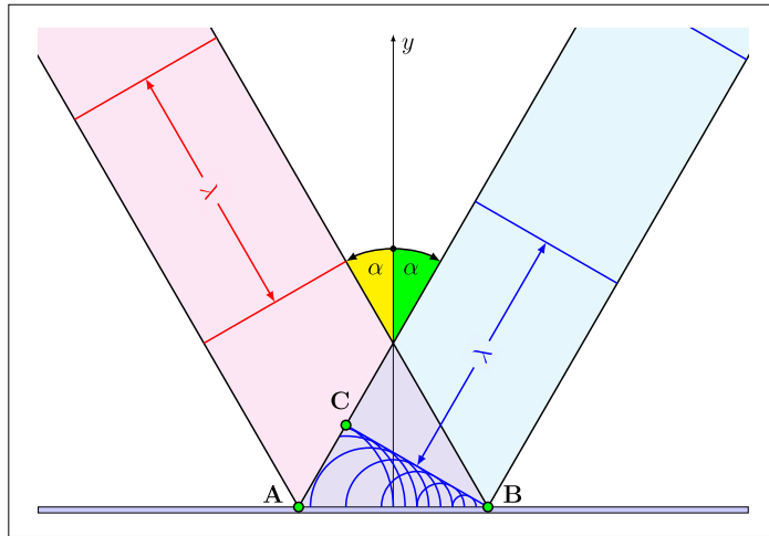
Abbildung 12.13: Huygens'sches Prinzip und Reflexionsgesetz.
