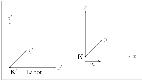
Abbildung 6.4: Laborsystem und Ruhesystem der bewegten Ladung.
