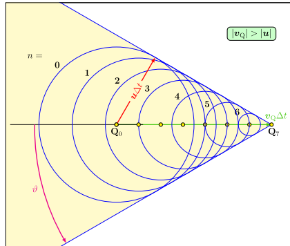
Abbildung 1.34: Schockwelle.
