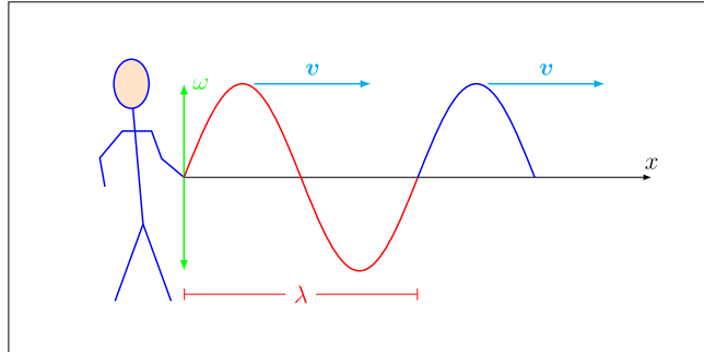
Abbildung 1.7: Harmonische Welle.
