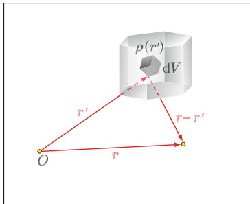
Abbildung 2.5: Ausgedehnte Ladungsverteilung.
