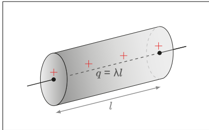
Abbildung 2.8: Berechnung des E-Feldes für einen unendlich langen, gleichmässig geladenen, Draht.
