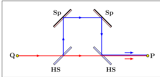
Abbildung 1.20: Aufteilung der von einer Quelle Q erzeugten Welle durch halbdurchlässige Spiegel HS und anschließende Interferenz im Punkt P . Sp sind nichtdurchlässige Spiegel.
