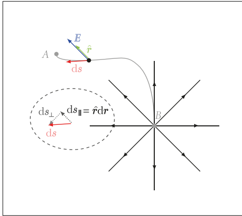
Abbildung 2.11: Berechnung des Potentials für eine Punktladung.
