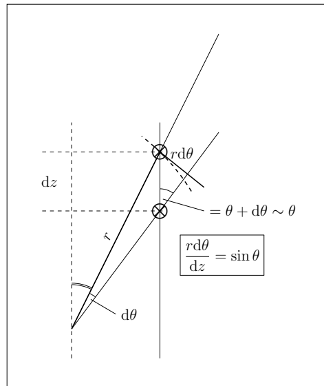
(c) Geometrie der Berechnung des Magnetfeldes.
