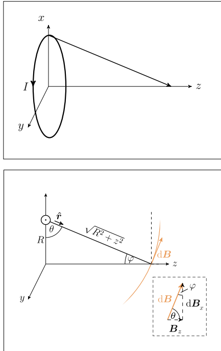
Abbildung 7.6: Feld eines kreisförmigen stromdurchflossenen Leiters.
