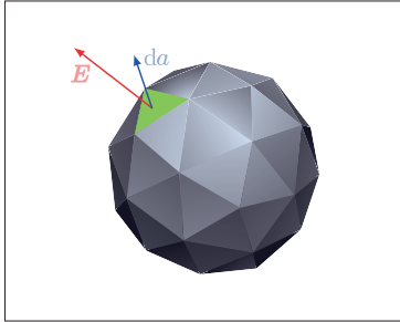
Abbildung 2.6: Geometrie zum Gauss'schen Gesetz.
