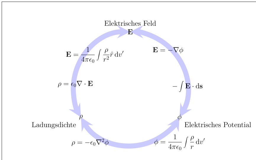
Abbildung 3.11: Beziehung zwischen Ladungsdichte \rho , elektrischem Feld \mathbf{E} und Potential \phi .
