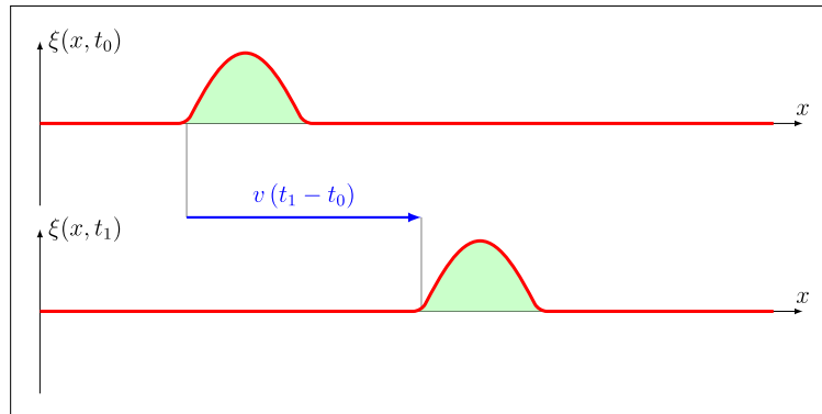
Abbildung 1.1: Ausbreitung einer Seilwelle.
