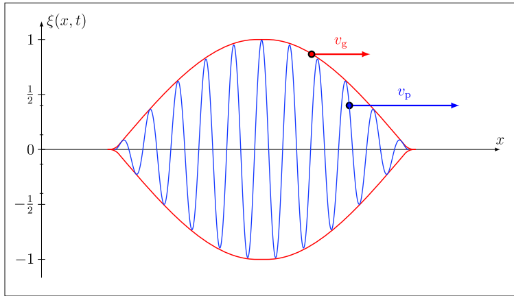
Abbildung 12.20: Wellenpaket.
