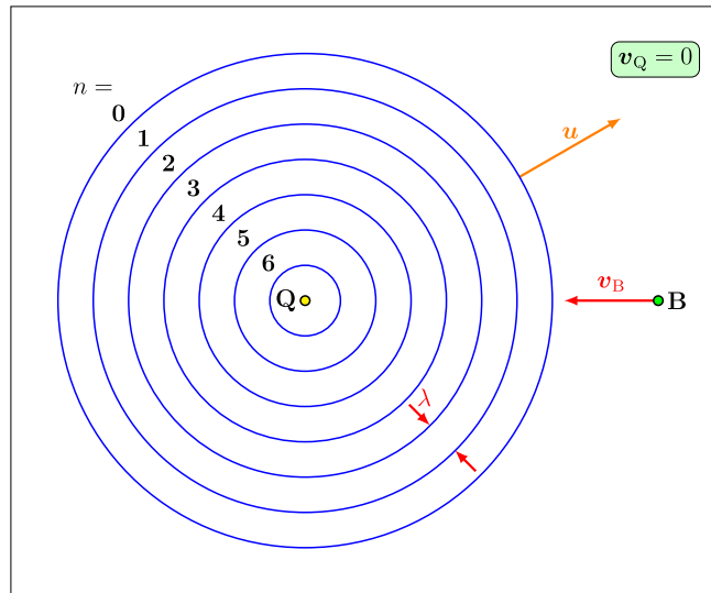
Abbildung 1.32: Dopplereffekt: Ruhende Quelle, bewegter Beobachter.
