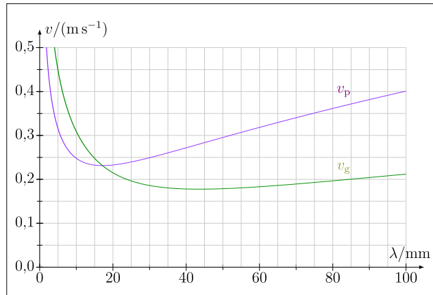
Abbildung 12.24: Gruppen- und Phasengeschwindigkeit als Funktion von \lambda bei \sigma = 0,072 N/m und h \rightarrow \infty .
