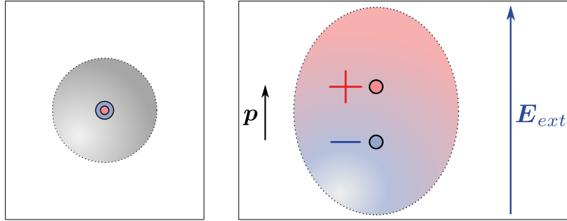
(a) Elektronen-Ladungsverteilung des Wasserstoffatoms im Grundzustand ohne äusseres Feld.
