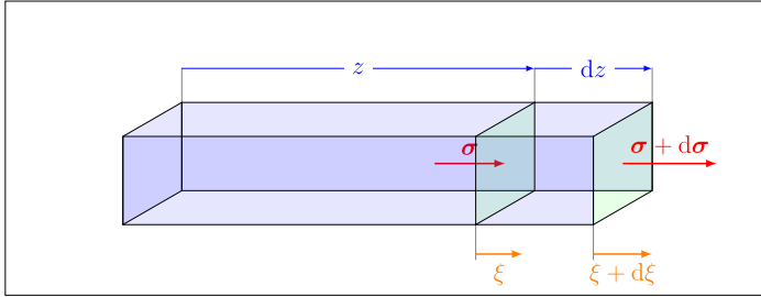
Abbildung 12.4: Zur Herleitung der Wellengleichung in einem Stab.
