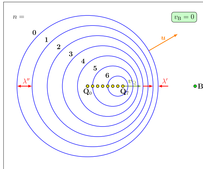
Abbildung 1.33: Dopplereffekt: Bewegte Quelle, ruhender Beobachter.
