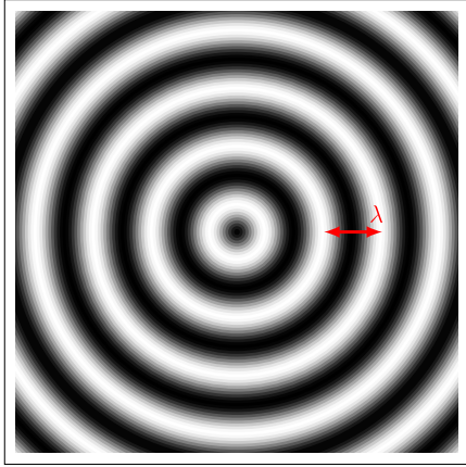
Abbildung 1.13: Longitudinale Kugelwellen.
