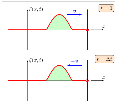
Abbildung 1.23: Reflexion eines Wellenberges am losen Ende.
