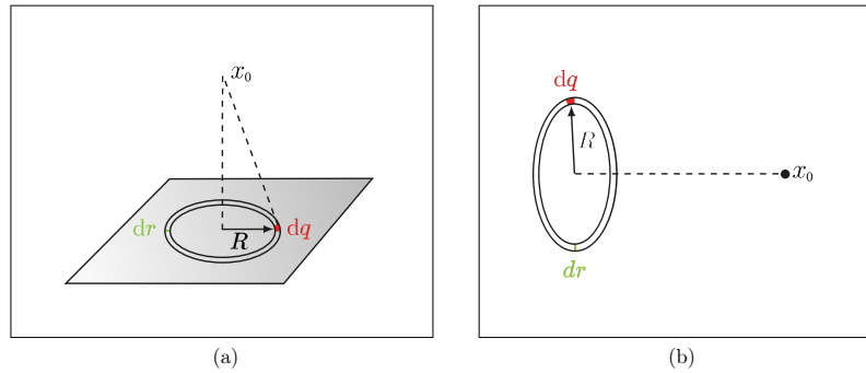
Abbildung 2.12: Berechnung des Potentials für eine Ringladung.
