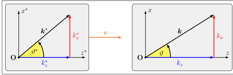
Abbildung 5.13: Relativistischer Dopplereffekt.
