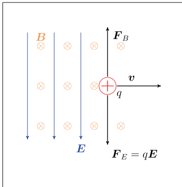
Abbildung 7.1: Kräfte auf eine Punktladung +q im elektrischen und magnetischen Feld, wobei \mathbf{E} \perp \mathbf{B} . Das Magnetfeld zeigt in die Papierebene.
