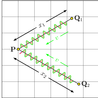
Abbildung 1.19: Gangunterschied.
