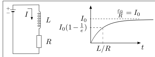
(b) Zeitverhalten nach Schliessen des Schaltkreises.
