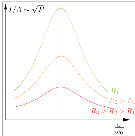
Abbildung 9.9: Resonanzkurven des RLC -Schaltkreises.
