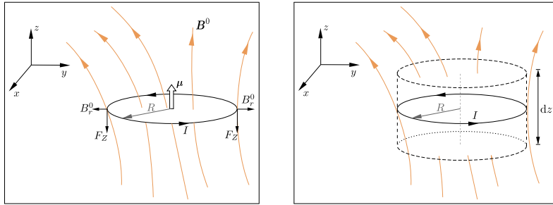
(a) Eine stromdurchflossene Leiterschleife im externen inhomogenen magnetischen Feld \mathbf{B}^0 . Die radiale Komponente des magnetischen Feldes B_r^0 erzeugen eine Lorentz-Kraft F_z , die auf die Schleife wirkt.
