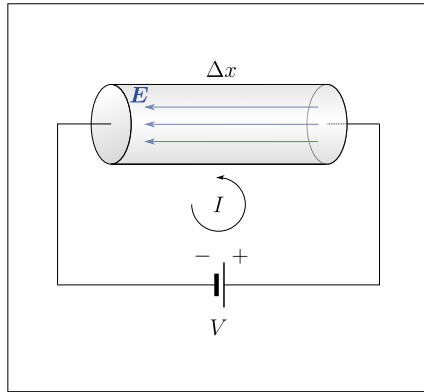
Abbildung 4.3: Eine mit einem Leiter verbundene Spannungsquelle.
