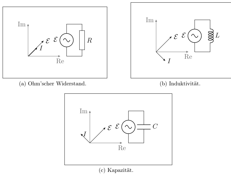
Abbildung 9.10: Relative Phasenlagen zu einer externen elektromotorischen Kraft für verschiedene Wechselstromkreise.
