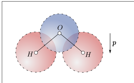
Abbildung 11.3: Das \text{H}_2\text{O} -Molekül hat ein permanentes Dipolmoment p = 6.2210^{-30} \text{ Cm} .
