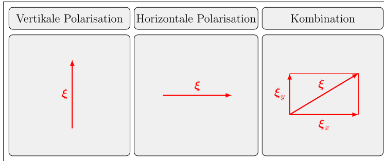
Abbildung 1.10: Lineare Polarisation.
