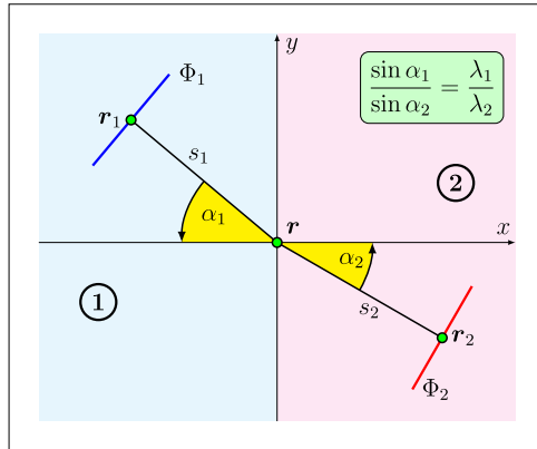
Abbildung 12.15: Fermat'sches Prinzip und Brechungsgesetz.
