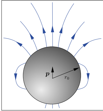
(a) Das äussere Feld einer homogen polarisierten Kugel mit Polarisationsdichte \mathbf{P} . Das Feld ist einem Dipol mit Dipolmoment \mathbf{p} = \frac{4\pi r_0}{3} \mathbf{P} äquivalent.
