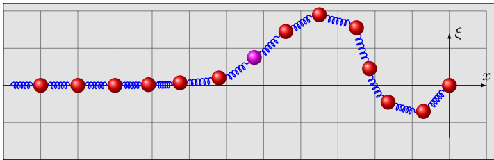
Abbildung 1.4: Transversale Wellen im Masse-Feder-System.
