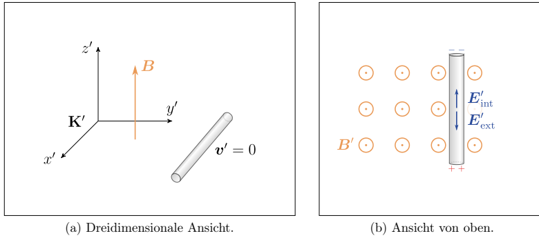
Abbildung 8.2: Situation von Abbildung 8.1 vom mitbewegten Koordinatensystem K' aus gesehen.
