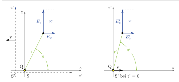
Abbildung 6.5: Elektrisches Feld im Ruhesystem der bewegten Ladung und im Laborsystem.
