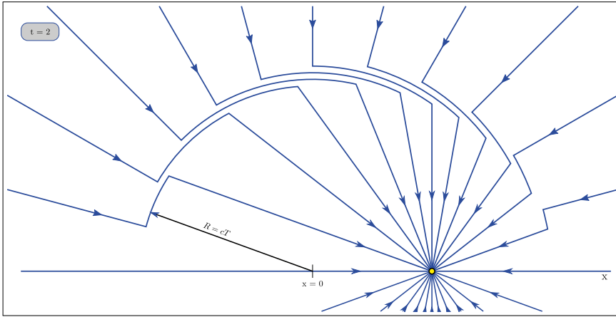
Abbildung 6.7: Feldlinien einer Punktladung, die zum Zeitpunkt t = 0 schlagartig beschleunigt wird und sich danach mit konstanter Geschwindigkeit fortbewegt.
