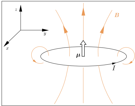
Abbildung 11.10: Feld einer Leiterschleife mit magnetischem Moment \mu .
