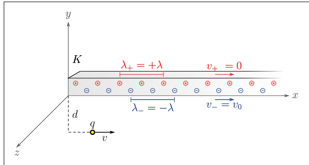
(a) Geometrie und Ladungsverteilung im Ruhesystem \mathbf{K} des Leiters (i. e. der Ionenrümpfe).
