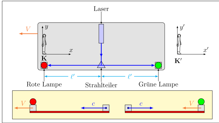
Abbildung 5.7: Der Tisch, wie er vom Beobachter K' gesehen wird. Der Beobachter sieht, dass die rote Lampe sich vom Lichtstrahl entfernt, und dass die grüne Lampe sich dem Lichtstrahl nähert.
