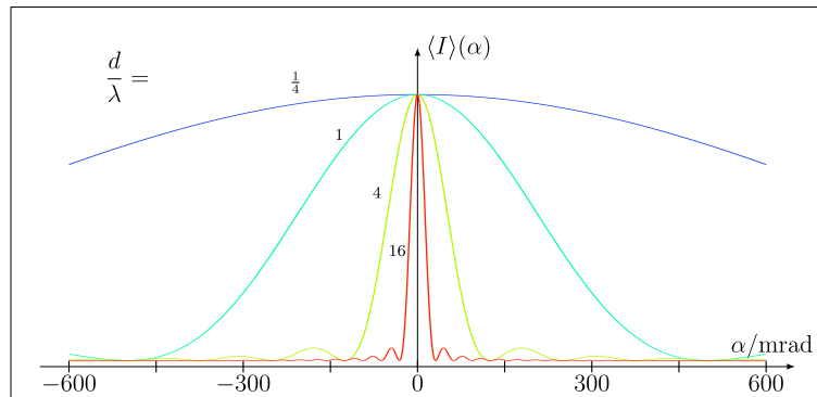
Abbildung 12.12: Beugung am Spalt.
