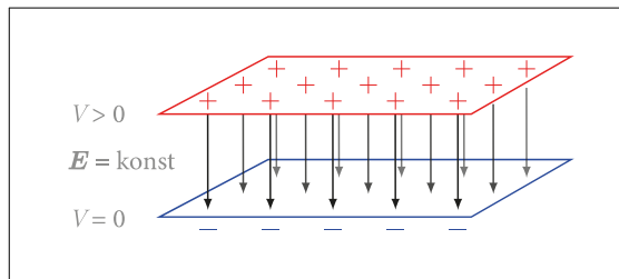
Abbildung 2.10: Feld und Potential eines Plattenkondensators.
