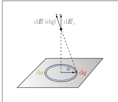
(b) Berechnung mit dem Coulomb'schen Gesetz.
