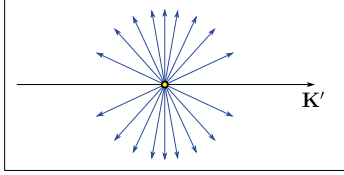
Abbildung 6.6: Feldlinien einer bewegten Ladung im Laborsystem \mathbf{K}' .
