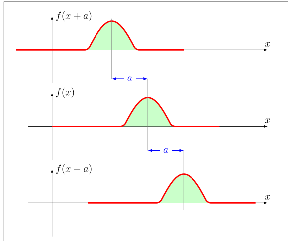
Abbildung 1.6: Translation eines Wellenbergs um a nach links (oberes Bild) bzw. um a nach rechts (unteres Bild).
