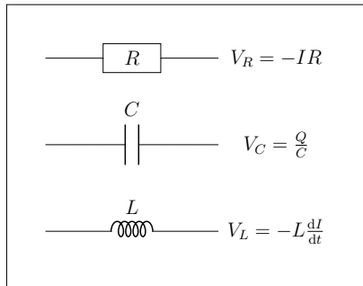
Abbildung 9.5: Zusammenfassung Spannungsabfälle.
